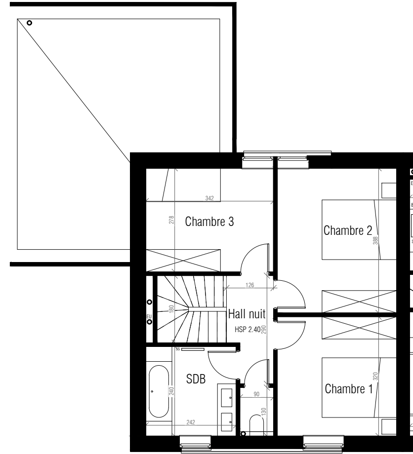
ÉTAGE
