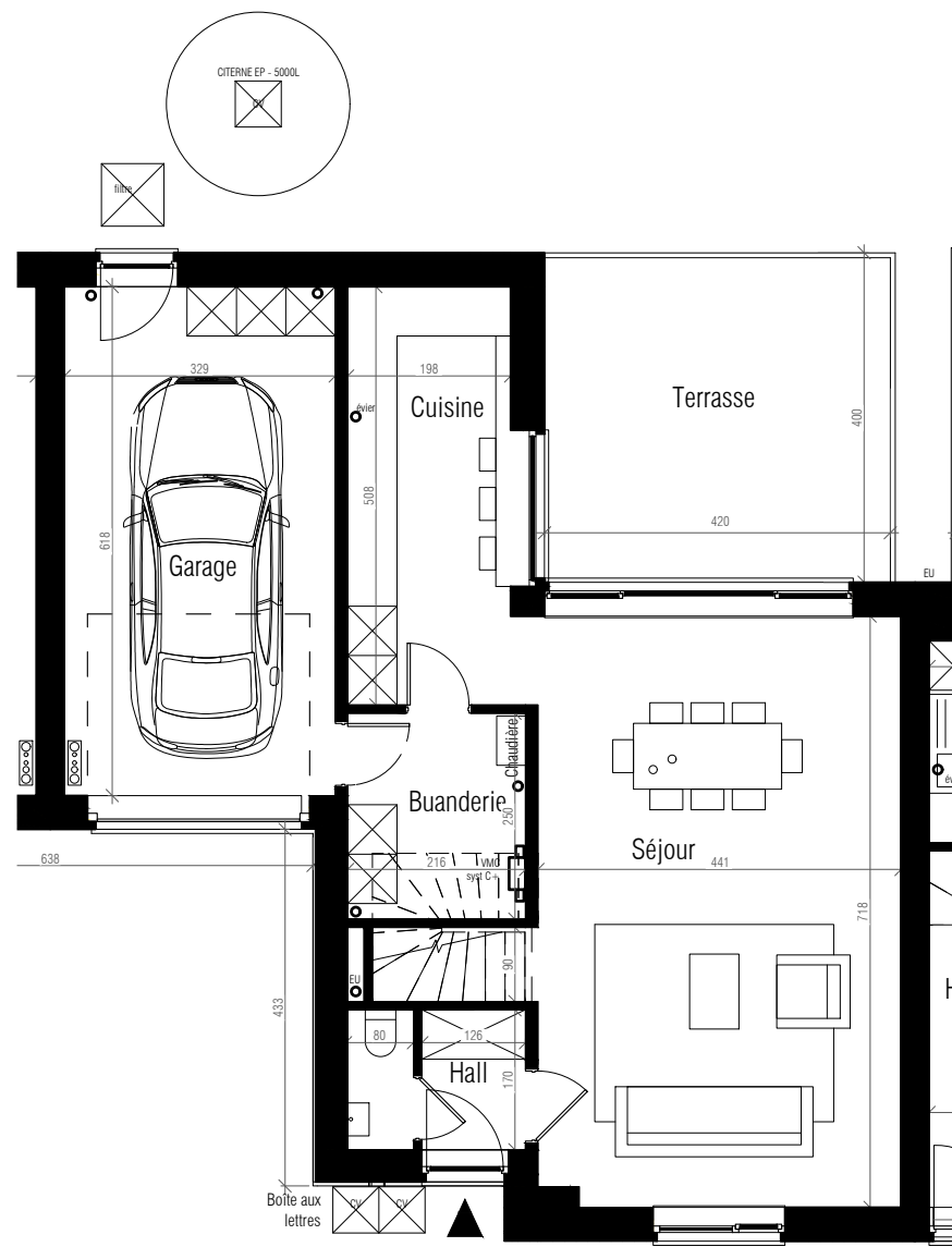
REZ-DE-CHAUSSÉE
